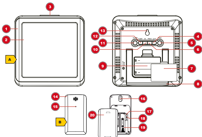
Рис. 1: Все части основного блока (наверху) и беспроводного внешнего датчика (внизу)
