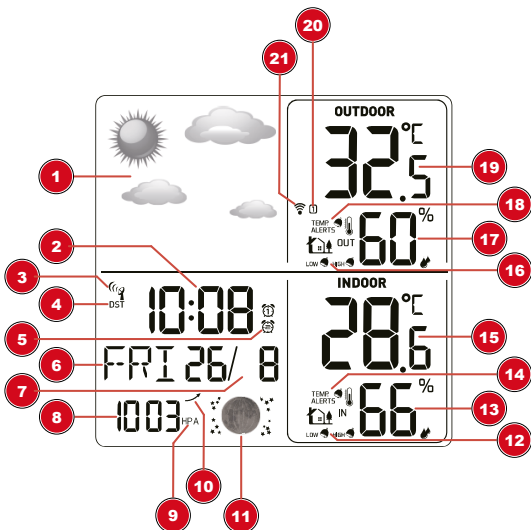
Рис. 2: Экран основного блока
