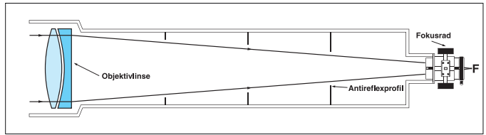
Abb. 61 Der optische Aufbau der Linsenteleskope beinhaltet ein optisches Design, bei dem das Licht von links kommend durch ein zweilinsiges Objektiv tritt und im Brennpunkt (F) fokussiert wird.
