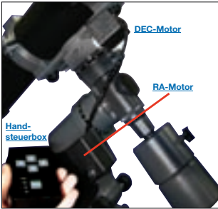
Abb. 65: Ein parallaktisch montiertes Teleskop mit nachgerüsteten Motoren
