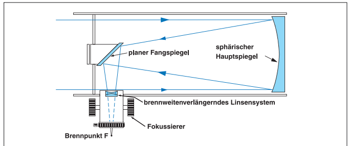
Abb. 62: Der optische Aufbau der Newton Spiegelteleskope beinhaltet ein brennweitenverlängerndes, achromatisches Linsensystem, das die Kombination von langer Brennweite und kurzem Tubus erlaubt.
