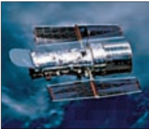
Abb. 1: Das Teleskop „Hubble“ im Orbit der Erde. Foto: NASA u. STScI
