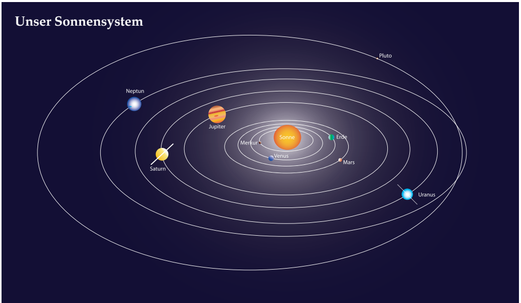
Abb. 14: Schematische Darstellung unseres Sonnensystems
